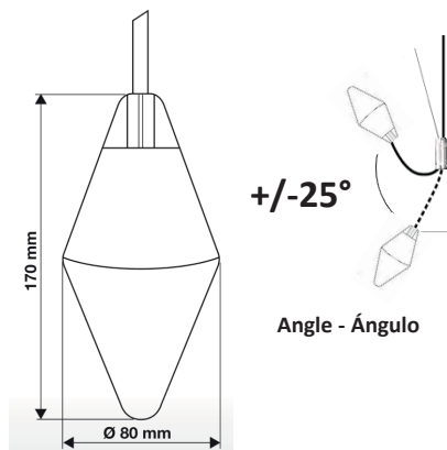
Dimension - Dimensión
